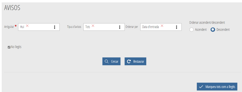
Figura 42. Pantalla d'avisos.
